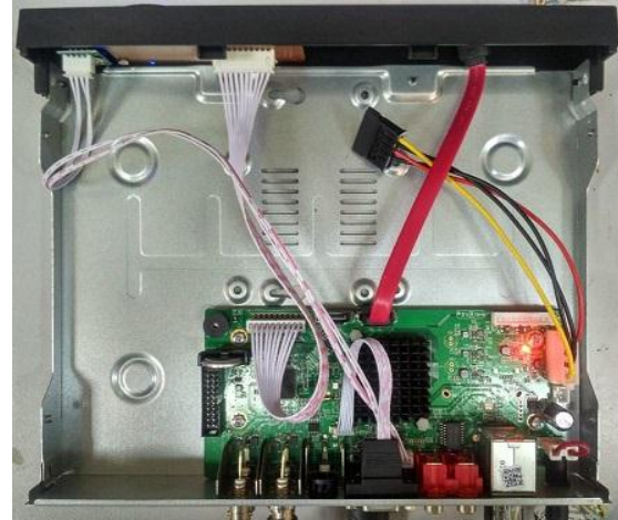
Внешний вид видеорегистратора без крышки.
